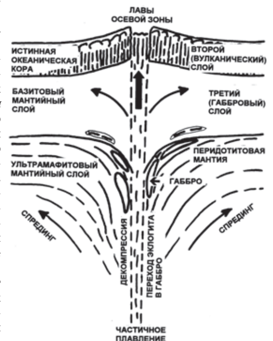
Рис. 2. Наглядная схема эволюции вещества мантии при его подъеме в зоне спрединга, принципиально отличающаяся от существующей канонической схемы (см. рис. 1) отсутствием гигантской осевой магматической камеры.
