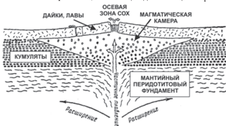
Рис. 1. Принципиальная каноническая схема образования океанического разреза и офиолитовой ассоциации (по Parrot, Ricou, 1976).
