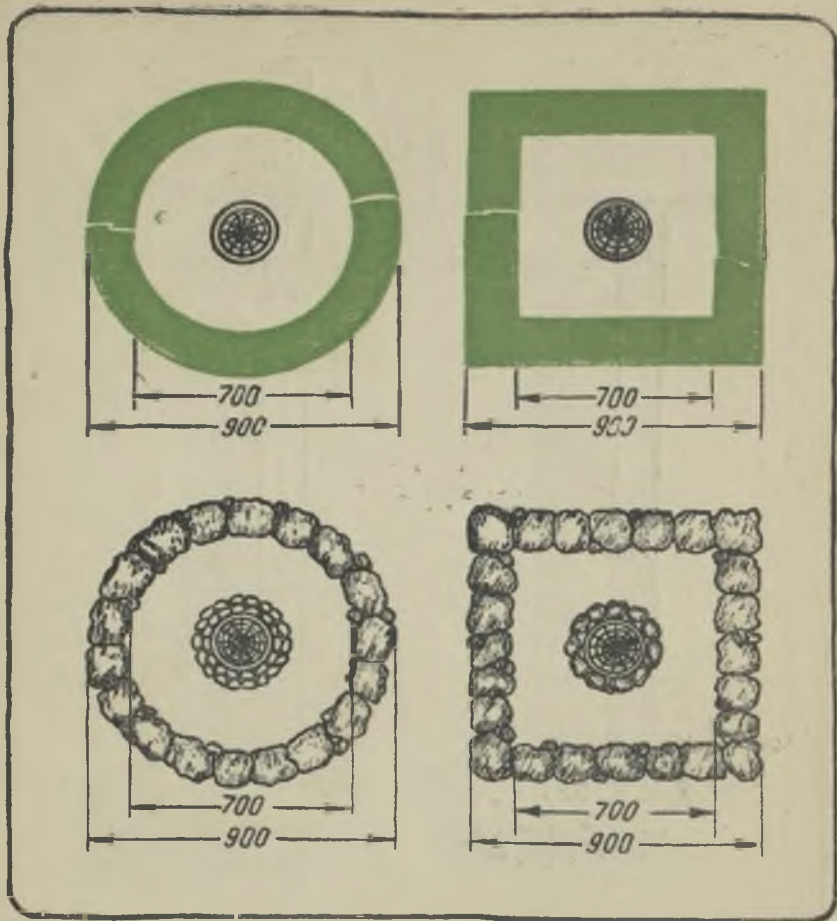
Разделка оснований столбов
