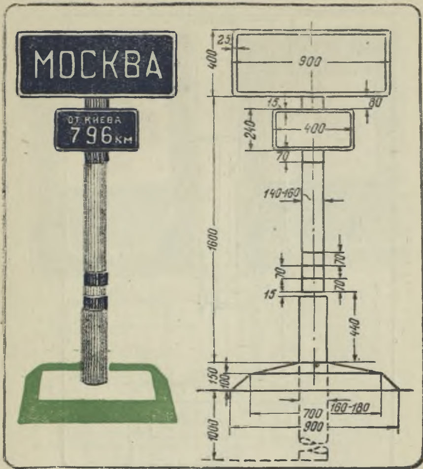
Чертеж щитка и столба для знака названия населенного пункта
