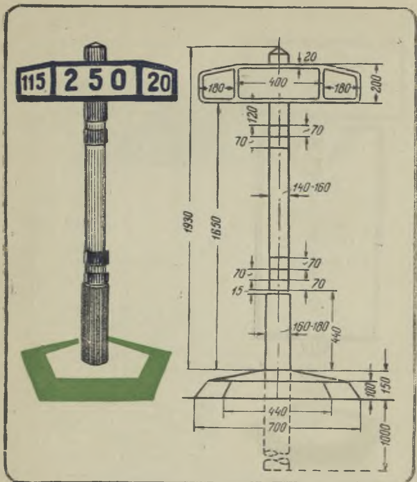
Чертеж установки километрового знака
