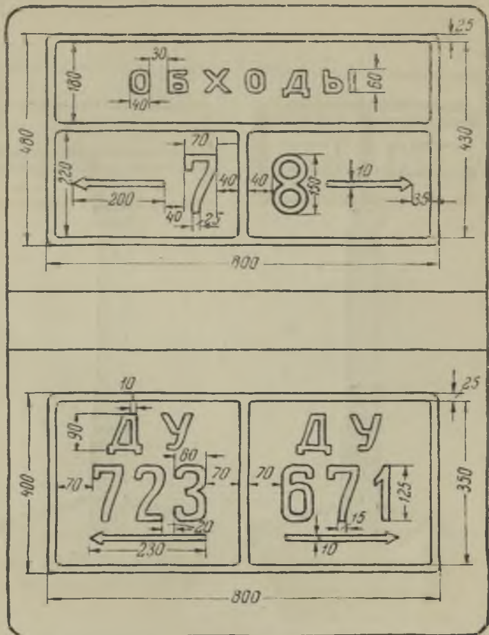
Чертеж знака границы обходов и участков
