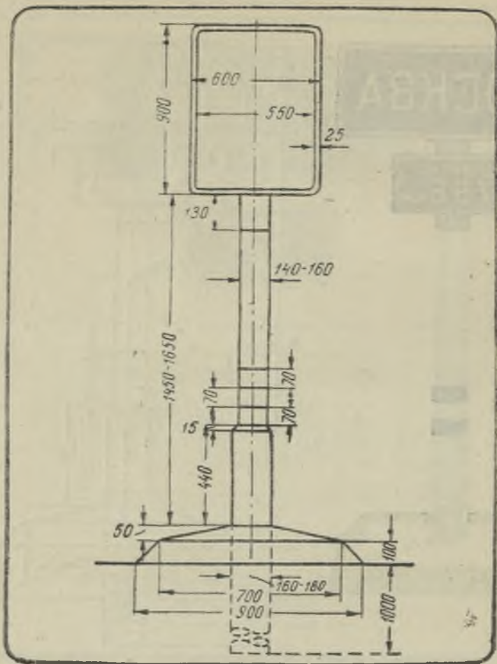
Чертеж щитка и столба для знака пункта первой помощи.
