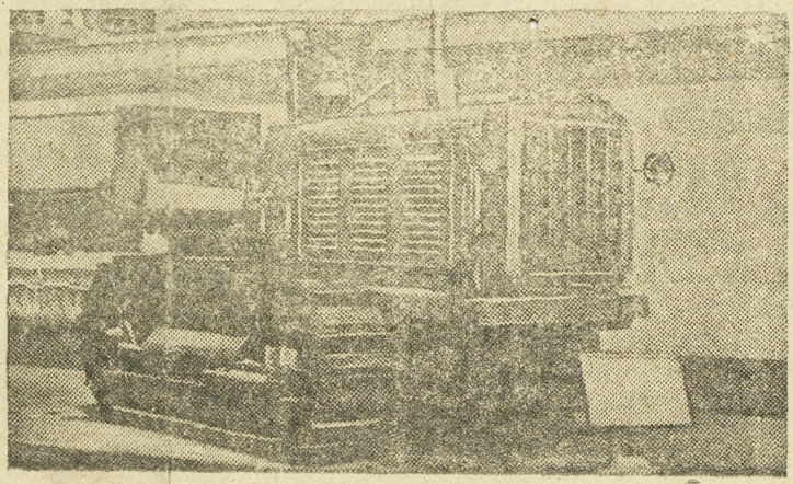
НА СНИМКЕ: новый экспонат павильона Механизации опытный образец гусеничного трактора ЧТЗ-Г-3465 с газогенераторной установкой НАТИ Г 34, работающей на древесном угле. Мощность двигателя 65 лошадиных сил. Фото С. Шмале. Фото Клише ТАСС.
