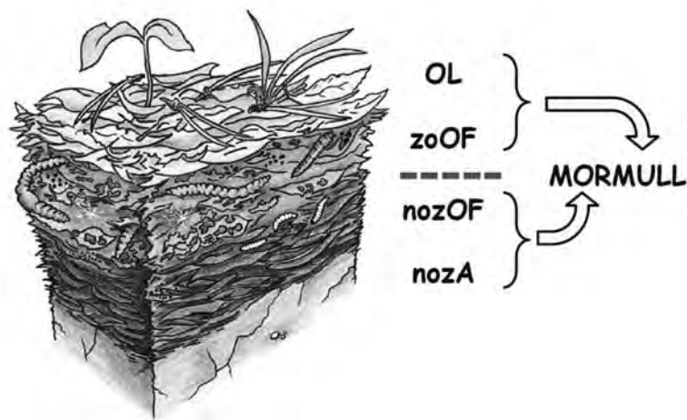
Схема строения форм гумуса из системы Мормюль: сверху зоогенные горизонты, внизу – неззоогенные
