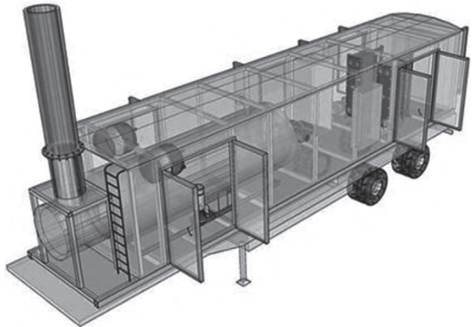
РИСУНОК 1. Схематичный вид передвижной котельной установки
