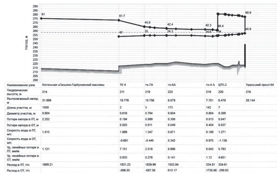
РИСУНОК 2. Котельная ГГМ-микрорайон ГГМ при аварийной ситуации на участке от ТК1а до ТК3а
