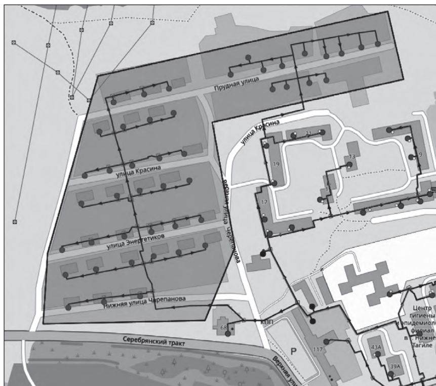
РИСУНОК 24. Зона перехода на индивидуальное теплоснабжение в микрорайоне индивидуальной жилой застройки Елизарова гора
