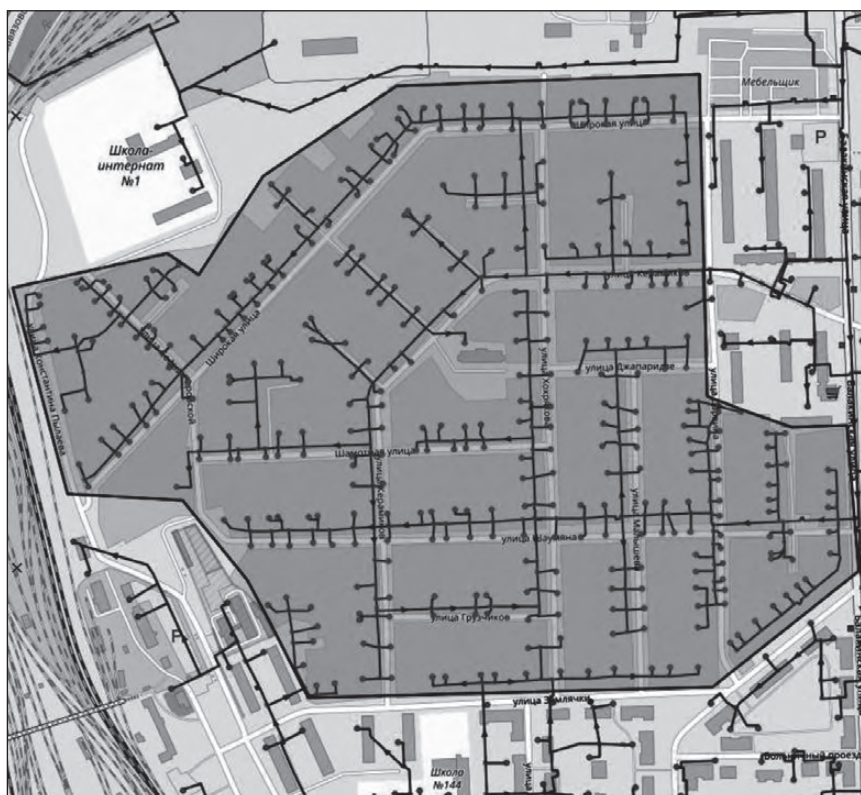
РИСУНОК 23. Зона перехода на индивидуальное теплоснабжение в микрорайоне индивидуальной жилой застройки Смычка
