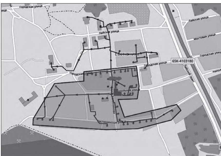
РИСУНОК 25. Зона перехода на индивидуальное теплоснабжение в микрорайоне индивидуальной жилой застройки поселок Евстюнина
