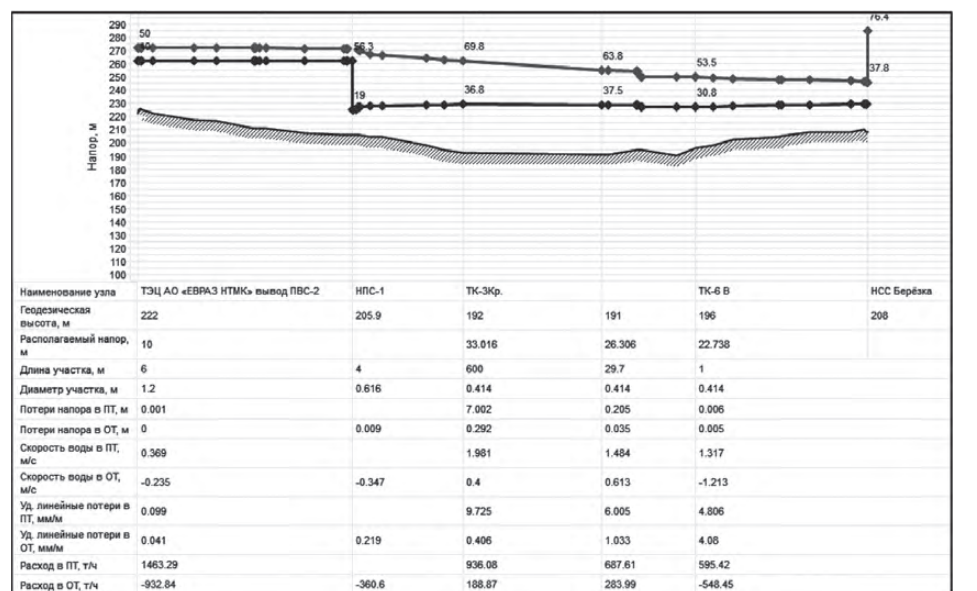
РИСУНОК 4. ТЭЦ АО «ЕВРАЗ НТМК» НПС-1- НСС «Березка» при аварийной ситуации на магистрали Ду600 от ТЭЦ ЕВРАЗ до ТК6в
