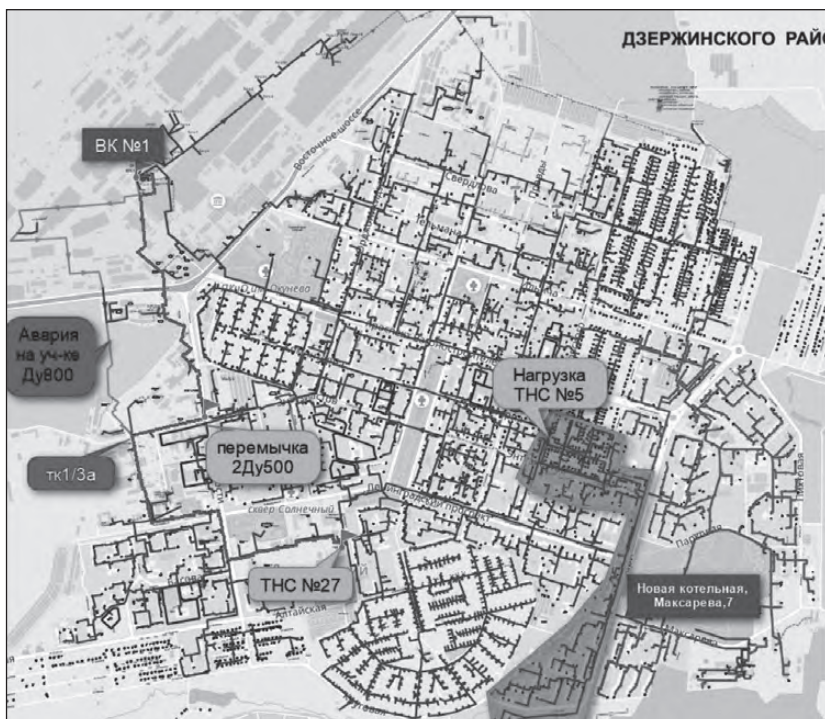
РИСУНОК 7. Смоделированная аварийная ситуация. Альтернативный путь движения теплоносителя
