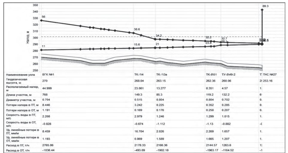
РИСУНОК 8. ВК № 1-ТНС № 27 при аварийной ситуации на магистрали Ду800 от ВК № 1 до ТК1/3а
