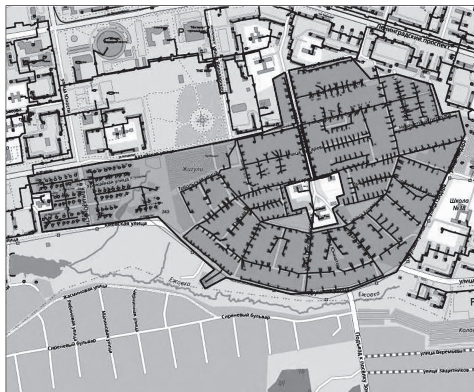
РИСУНОК 27. Зона перехода на индивидуальное теплоснабжение в микрорайоне индивидуальной жилой застройки «Девятый поселок»
