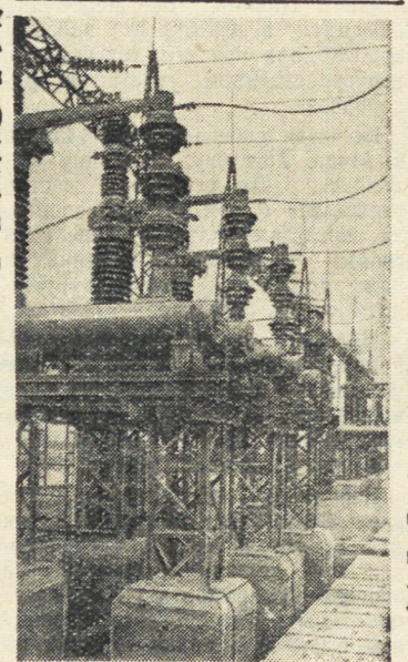
Эстонская ССР. Строительство Нарвской ГЭС вступило в предпусковой период. Скоро первая турбина даст ток.
