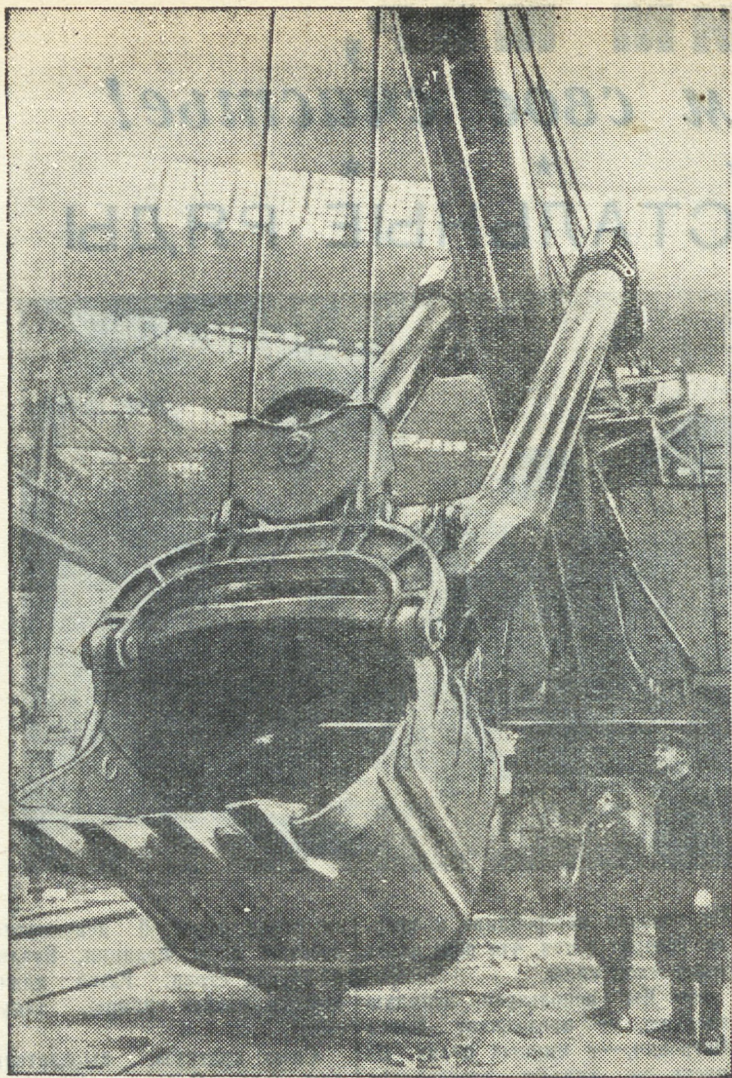
Ковш нового шестикубового экскаватора.
