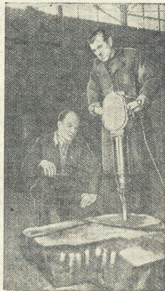
Сотрудники Всесоюзного научно-исследовательского института строительного и дорожного машиностроения Н. М. Батуевым и Д. С. Федосеевым создан ручной электромотол для разрушения мерзлого грунта и бетона.
