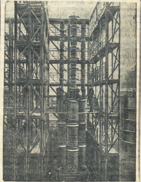
Завод «Уралэлектроаппарат» изготавливает мощный выключатель на 400 тысяч вольт для Куйбышевской ГЭС и линии электропередач Куйбышев — Москва.
