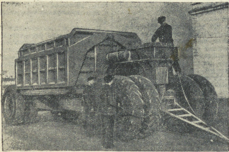
Белорусская ССР. Минский автозавод выпустил два опытных прицепа-самосвала. Кузов прицепа может разгружаться на обе стороны с помощью гидравлического механизма. НА СНИМКЕ: новый 40-тонный прицеп-самосвал «МАЗ-5210». Фото М. Микевича (Фотохроника ТАСС).
