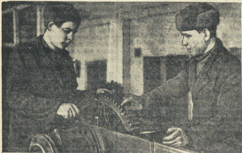
НА СНИМКЕ: молодой механизатор-стахановец Зайковской МТС Петр Тютин и кандидат в народные заседатели коммунист И. К. Уноров регулируют дифер и промежуточную передачу трактора. Снимок И. Исакова.
