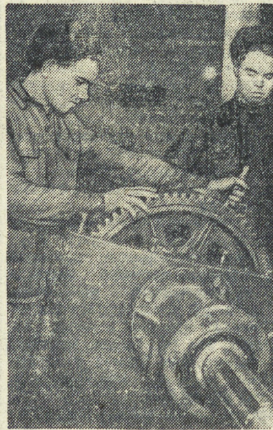
Молодые трактористы Камышловской МТС Василий Шырыкалов и Александр Булатов обязались ко дню выборов в Верховный Совет РСФСР отремонтировать задние мосты ко всем тракторам. Сейчас они ежедневно выполняют задания на 150 процентов.
