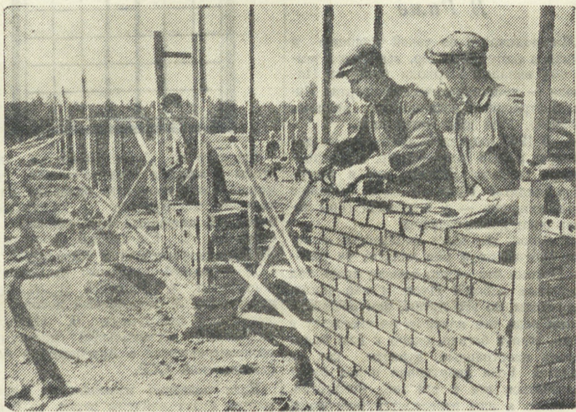
В колхозе «Заря», Ачитского района, строится новая молочно-товарная ферма. На ее территории будут сооружены пять коровников, маслозавод, 6 бетонированных силосных ям и телятники. Сейчас воздвигаются столбы кирпичной кладки, прокладывается водопровод. Строительством ведет прораб Владимир Вишняков (первый справа), учащийся Свердловского строительного техникума.
