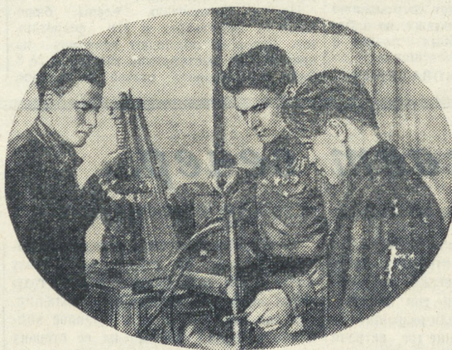
Активные участники помощи промышленности студенты механического факультета (слева направо): В. Кривошея, Ю. Маслов, А. Шаламов за установкой для точной сварки экспериментально проверяют данные доклада Ю. Маслова «Контактная сварка в машиностроении».
