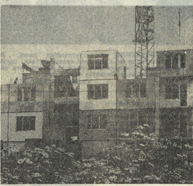
Этаж — за один день , в таком темпе сооружаются сейчас жилые дома из объемных блоков в некоторых микрорайонах Минска. Объемные блоки выпускает городской домостроительный комбинат № 3. Каждый блок представляет собой почти готовую комнату или санитарно-техническое помещение. Оно 75 процентов отделочных работ в изготовленных блоках производится на комбинате. Если на монтаж 60-квартирного крупнопанельного дома затрачивается 25 дней (без учета нулевого цикла строительства), то такой же дом из объемных блоков монтируется за 11 дней. Снимок АПН.
