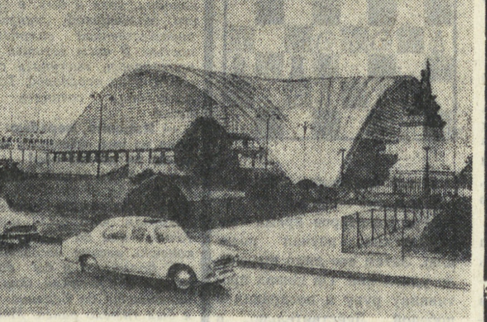
Париж. Французский национальный центр индустрии и техники (на снимке) размещается в здании оригинальной конструкции. Три стеклянных треугольника покрывают трюны, сходящиеся в одной точке сводами, с 218-метровым пролетом, имеющим опоры только в трех точках. Здание предназначается для больших французских и международных выставок. Снимок АФП—ТАСС.
