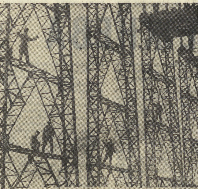
Ингури ГЭС строится. Снимок Г. Кинквадзе и С. Тевзадзе.
