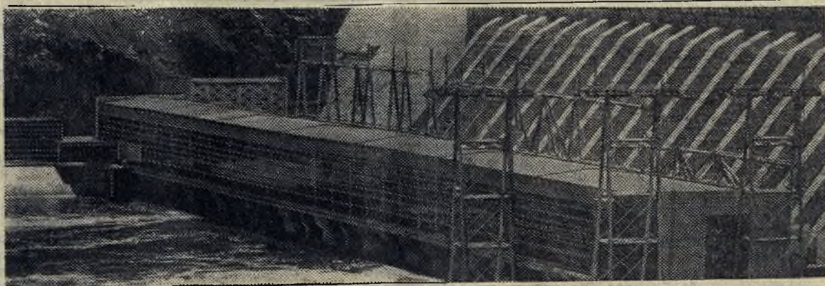
Дивногорск. Скоро Государственная комиссия подпишет акт о сдаче крупнейшей в мире Красноярской ГЭС в промышленную эксплуатацию. Будет подведен итог многомесячных наблюдений за работой основных сооружений, станции и ее оборудования. Здесь установлено 12 гидроагрегатов, мощность каждого из них 500 тысяч киловатт. (Фотохроника ТАСС).
