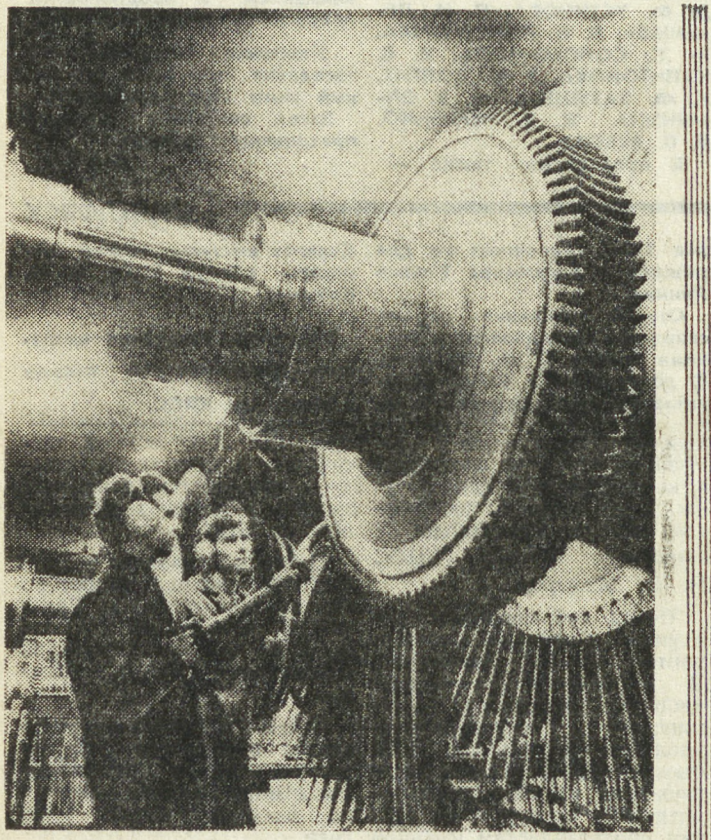
УКРАИНСКАЯ ССР. На Харьковском турбинном заводе имени Кирова, поставившем свою продукцию странам СЭВ, заканчивается изготовление турбины мощностью 220 тысяч киловатт для атомной электростанции «Норд-2» в ГДР. На снимке: члены бригады коммунистического труда слесари-сборщики В. Шевченко (справа) и Ю. Кривоноз с сборной ротора низкого давления турбины для ГДР. Снимок М. ТУРА. Фотохроника ТАСС.
