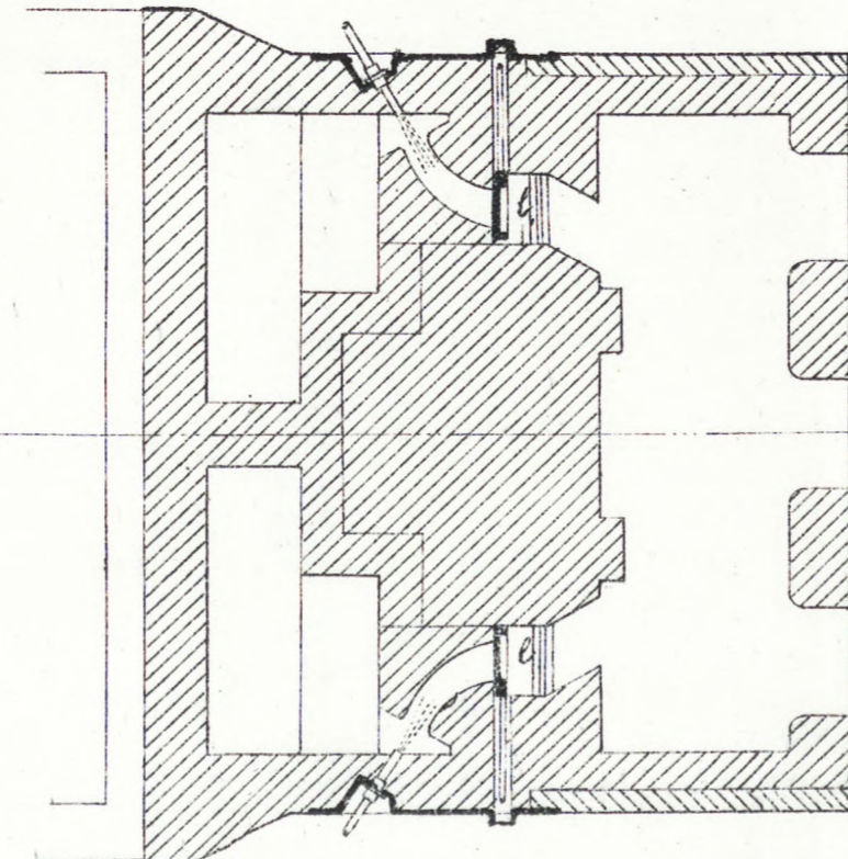
Ф.9. Разрѣзъ по линіи Г Г.
