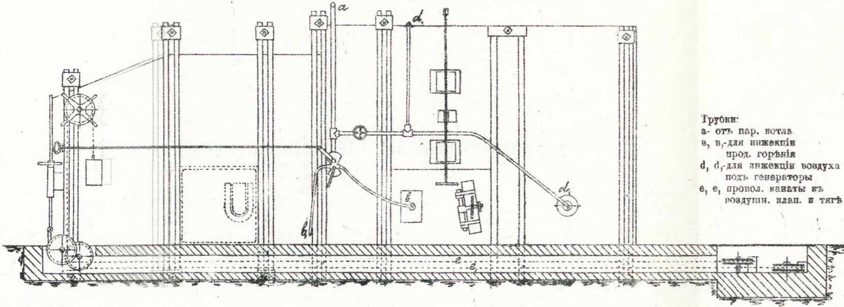
Ф.2. Разрѣзъ по линіи А А А А.
