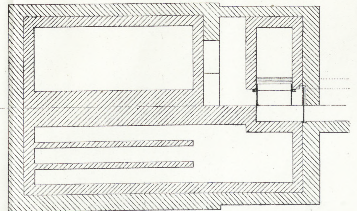
Ф.10. Разрѣзъ по линіи Н Н.
