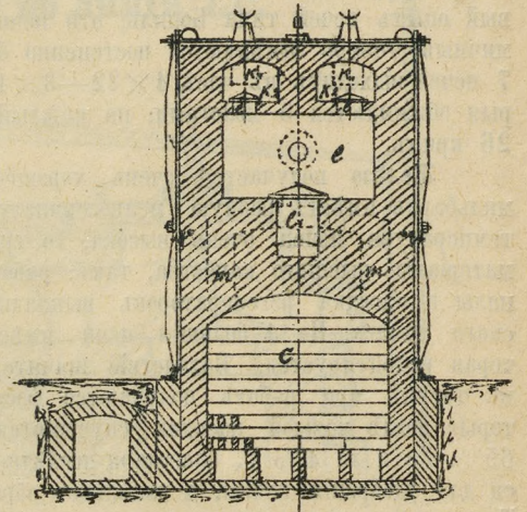
Ф 3. Разрѣзъ по ГЕ.
