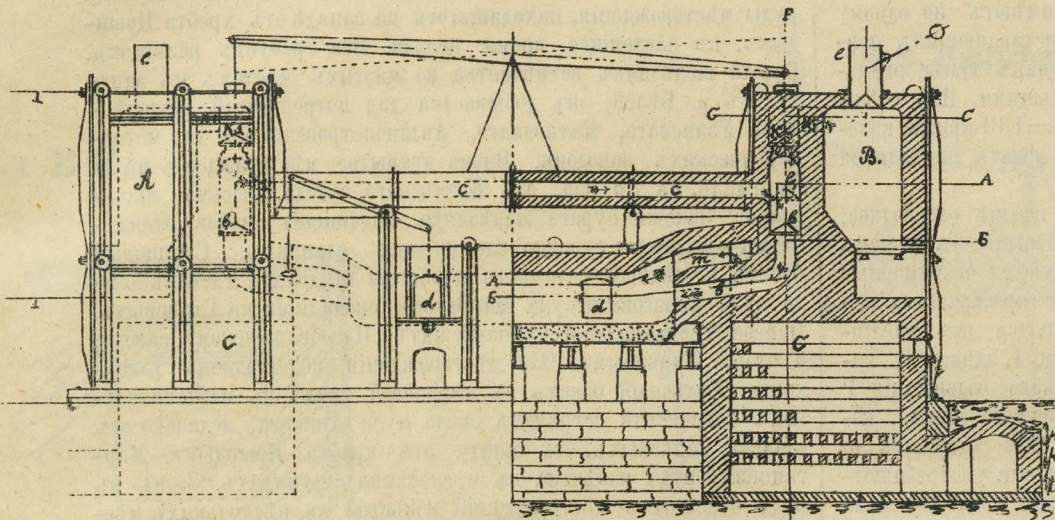
Разрѣзъ по БВ. Ф 2. Разрѣзъ по АА.
