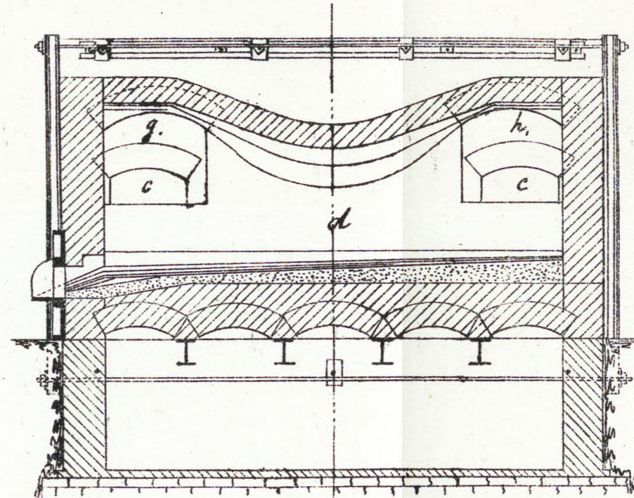
Разрѣзъ по линіи В С С.
