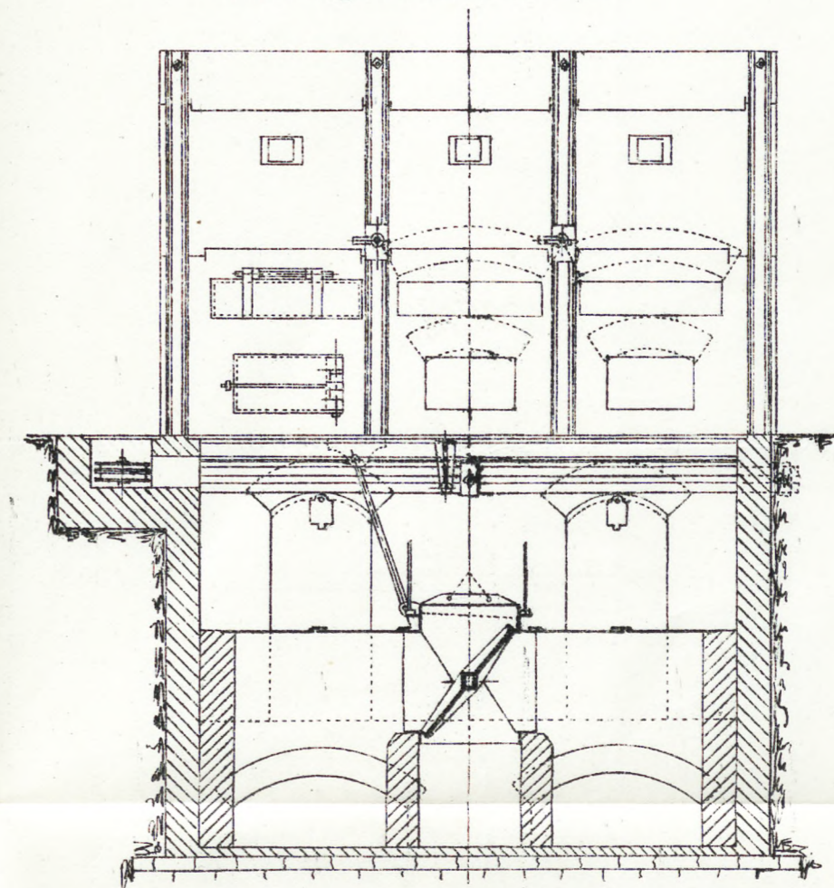
Ф.8. Разрѣзъ по линіи Д Д.
