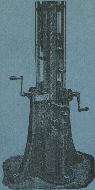
Машина для испытанія ударовъ системы Ш. Фремона.
