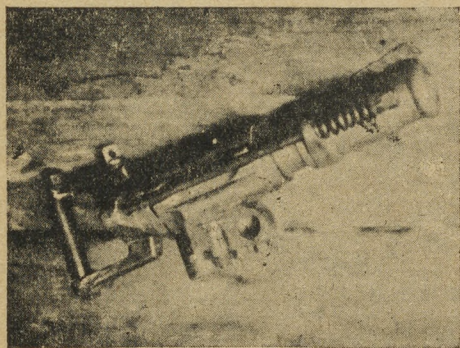
Перфоратор в собранном виде. Состоит из 30 деталей. Вес около 30 кгр.
