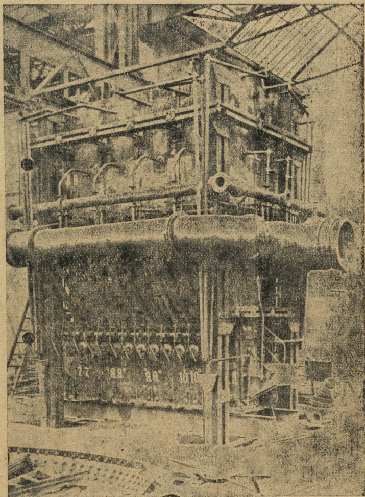
Карабаш. Ватержакет — специальная печь для плавки меди.
