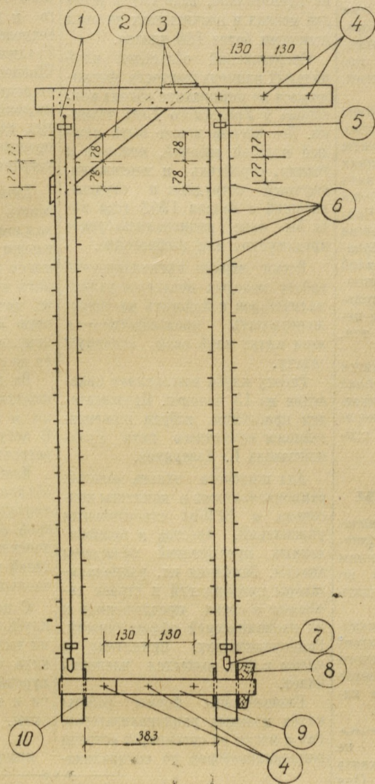
1 — доски 40×60 мм; 2 — подкос 40×60 мм; 3 — гвозди; 4 — болты \varnothing 12 l=80 мм; 5 — планка для отвеса; 6 — риски; 7 — отвес; 8 — клин; 9 — металлический хомут из полосовой стали 40×4 мм; 10 — фанерная прокладка 150×50×3 мм.
