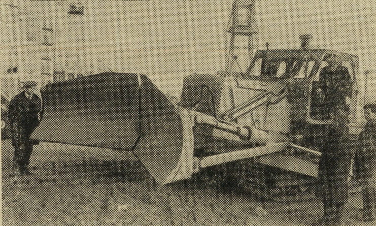
На снимке: один из экспонатов выставки — бульдозер с шарнирно-поворотным отвалом на тракторе «Т-100 МГП», предназначенный для планировочных работ на дорожном и жилищном строительстве. Угол поворота отвала вперед и назад — 25 градусов. Управление отвалом — гидравлическое. Фото Н. Кулешова. Фотохроника ТАСС.
