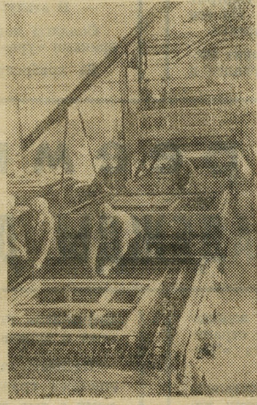
ХАБАРОВСК. Выпуск керамзитобетонных панелей на полуавтоматической конвейерной линии с бункерами и предварительным электроподогревом освоили хабаровские домостроители.
