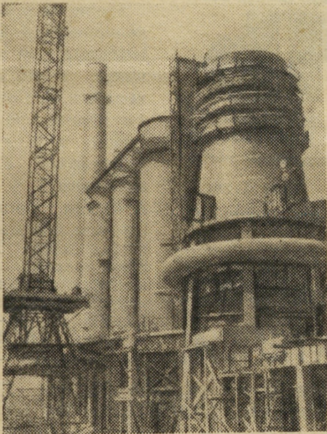
Народная Республика Болгария. Кремиковский металлургический комбинат. Вид на доменную печь.
