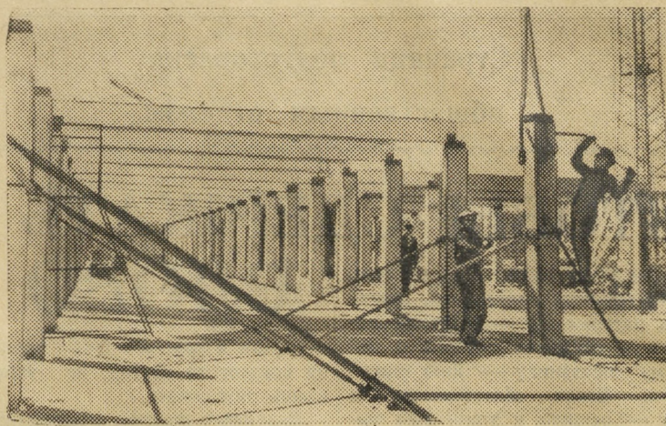
На снимке: монтаж колонн первого этажа школы из крупных панелей.
