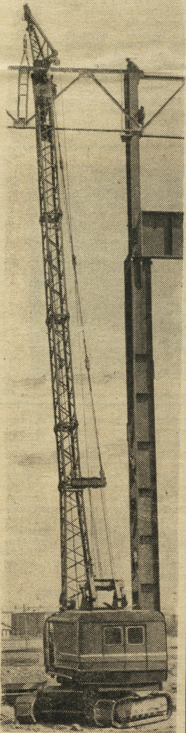
На строительстве высотных пролетов второй очереди ЦСМК. Фото А. Грахова.
