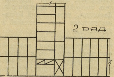
Примыкание стен при кладке в 2×1,5 кирпича.
