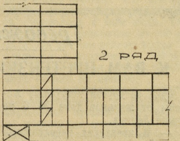
Перевязка углов при толщине стены в два кирпича.
