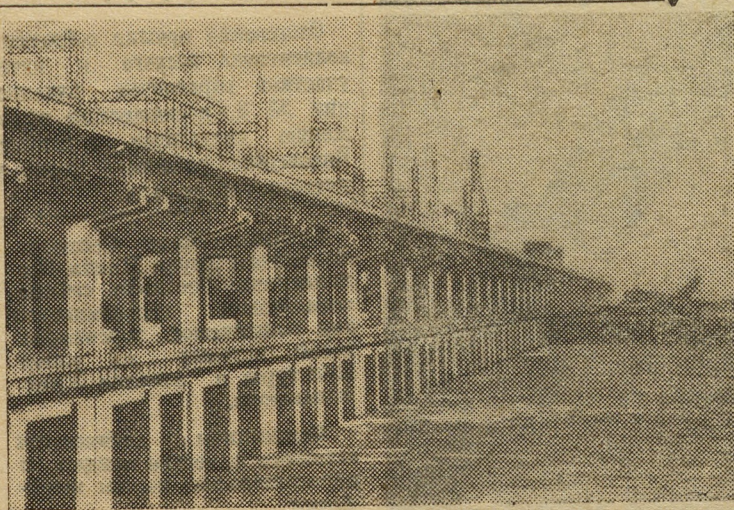
Крупнейшая в мире Сталинградская ГЭС. Фото С. Курунина. Фотохроника ТАСС.
