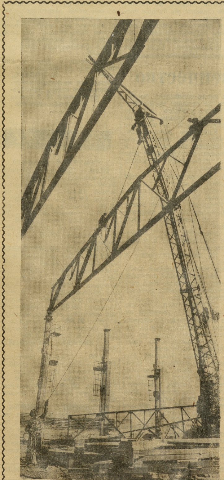
Напряженная работа кипит на строительстве цеха сварных машиностроительных конструкций. Сейчас здесь хозяйничают монтажники треста «Уралстальконструкция». Под руководством опытного прораба Михаила Владимировича Корякина они ведут монтаж каркаса самого крупного в Европе нового цеха.
