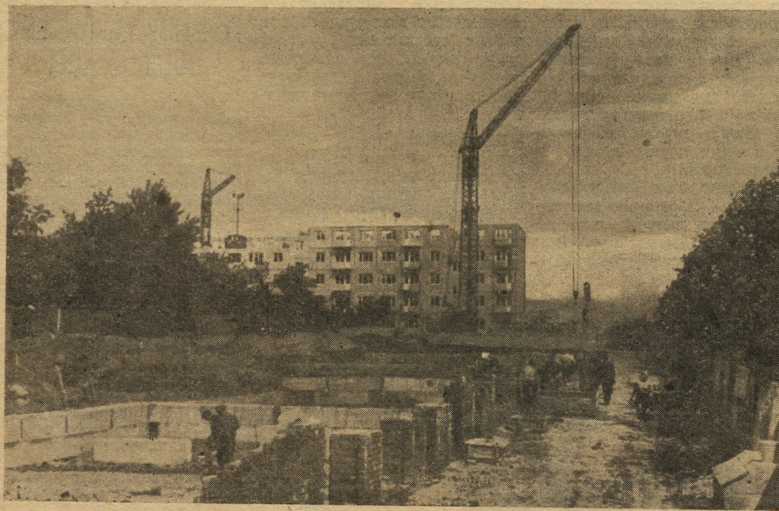
Строительство квартала № 10 (на углу улиц Восточной и Декабристов). Монтаж крупнопанельных домов здесь ведут бригады тт. Автаева и Кишки из первого управления треста № 33.
