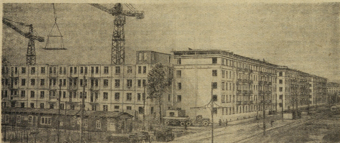
ЛЕНИНГРАД. Строительство домов в 30-м квартале Малой Охты из крупных панелей, изготовленных на предприятиях треста «Стройдеталь-81».
