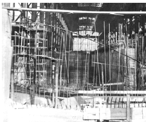
Фундаменты печей. 1967 год
