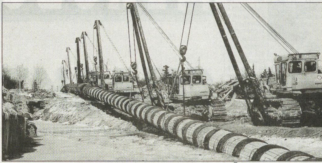
По этому дюкеру уже идет газ.
