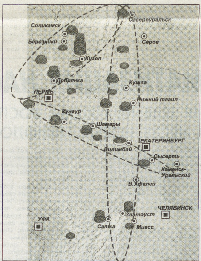
Среднеуральская сейсмогенная зона. Выделены Западно-Уральское, Средне-Уральское и Восточно-Уральское сейсмогенные направления. Диаметр дисков — энергия землетрясения: 6 и более, от 5 до 6 и менее 5, соответственно. Количество дисков — количество землетрясений.
