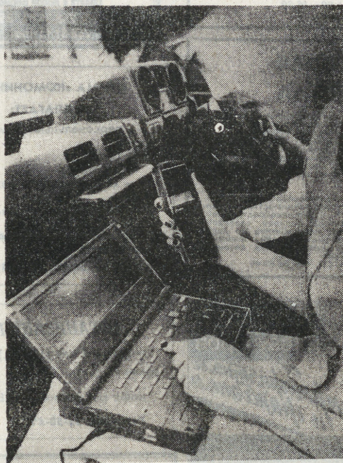
ЯПОНИЯ. Всемирно известная корпорация «Сони» изобрела новый портативный факсимильный аппарат, не требующий специальной бумаги. Текст любого послания набирается на экране аппарата и через телефонную связь передается адресату. Вес аппарата — 1,5 кг. Стоимость около 1500 долларов. Предполагается, что новые факсимильные аппараты поступят в продажу в июне этого года.
