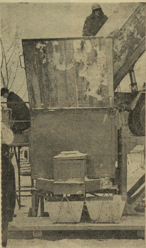
На фотографии вы видите приемный бункер, который установлен на доме треста «Гражданстрой» по улице Крауля. В бункере установлен шнек, перемешивающий раствор. Затем небольшими дозами раствор подается в металлические ящики, которые доставляются на рабочее место. В ближайшем будущем такой бункер будет установлен и на объектах домостроительного комбината.
