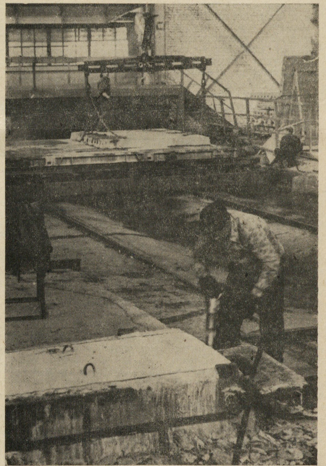
В цехе № 6 завода ЖБИ. Фото В. Калимасова.
