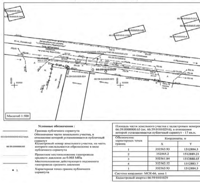
СХЕМА расположения границ публичного сервитута на часть земельного участка с кадастровым номером 66:59:0000000:65 (кад. № 66:59:0101029:6) на кадастровом плане территории в кадастровом квартале 66:59:0101029 для размещения газопровода среднего давления до границы земельного участка по адресу: г. Полевской, ул. Совхозная (кад. № 66:59:0101029:825)
