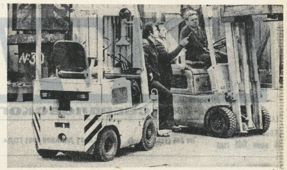
Маневренные, удобные, сильные — такую характеристику дают специалисты и водители двух моделей грузоподъемных машин, созданных коллективом головного специального конструкторского бюро по автомобильной технике в Свердловске. Успешно завершены комплекс заводских и государственных испытаний одностопного и двухтонного автопогрузчиков. Диапазон применения новых машин широк: они могут заезжать прямо в вагон или железнодорожный контейнер и выполнять там погрузочно-разгрузочные операции. Благодаря своим небольшим размерам незаменимы также на внутризаводских и внутрицеховых перевозках, в аэро- и морских портах. Конструкторы «научили» машины умело «работать» с самыми разнообразными по форме грузами: бочками, пушками, ящиками. Широкое внедрение новых машин сулит большие выгоды народному хозяйству страны, их эксплуатация обходится в полтора раза дешевле ныне применяющихся элеваторов. НА СНИМКЕ: новые машины. Фото В. КРИШТУЛА. (Фотокоринка ТАСС).
