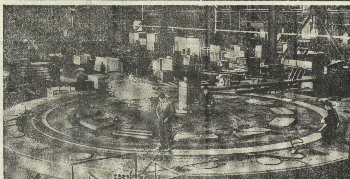
Во многих странах мира известны шагающие экскаваторы. Они хорошо зарекомендовали себя в карьерных выработках. Сейчас уральшанцы, выпускающие их, собирают очередную машину марки ЭП-20-90. Слесари-сборщики из бригады В. Ольханова завершают сборку отдельных узлов экскаватора. Фото В. ЯКУБОВА.
