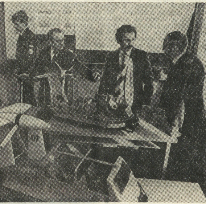
Латвийская ССР. Вездеход на воздушной подушке разработан в студенческом конструкторском бюро Рыжского Краснознаменного института инженеров гражданский авиации имени Ленинского комсомола. Новая машина свободно движется по тундре, болоту, речной гряде. По мнению кол-
