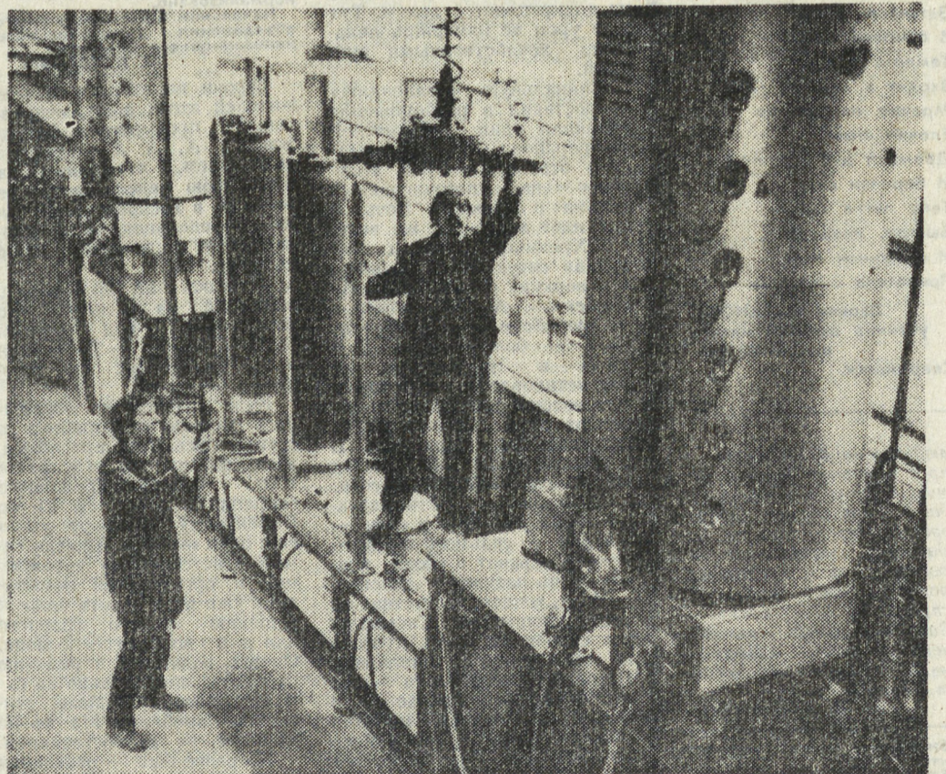
На Кировградском заводе твердых сплавов идет сборка установки нанесения многослойных инертностойких покрытий на многоразовые неперекаливаемые пластины. С внедрением в производство такой установки ресурс работы выпускаемого режущего инструмента увеличился в два-три раза. Сборку и наладку установки ведут наладчики Виктор Бурлаков и Александр Сырвачев. К концу текущего года наладчик обзавелся первой пробной продукцией. НА СНИМКЕ: на сборке установки наладчики В. Бурлаков и А. Сырвачев. Фото Л. БАРАНОВА.
