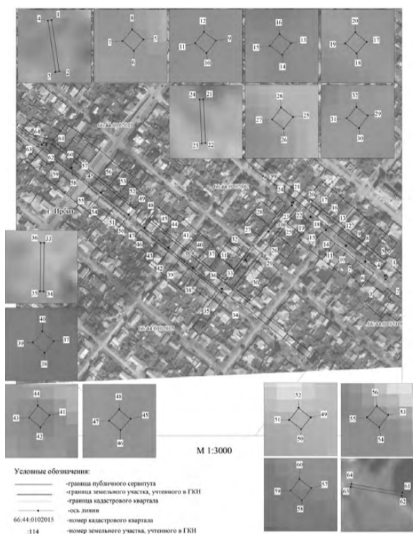
Публичный сервитут ВЛ-6 кВ на ж/б опорах от ТП 3105 до ТП 3106 Схема расположения границ публичного сервитута
