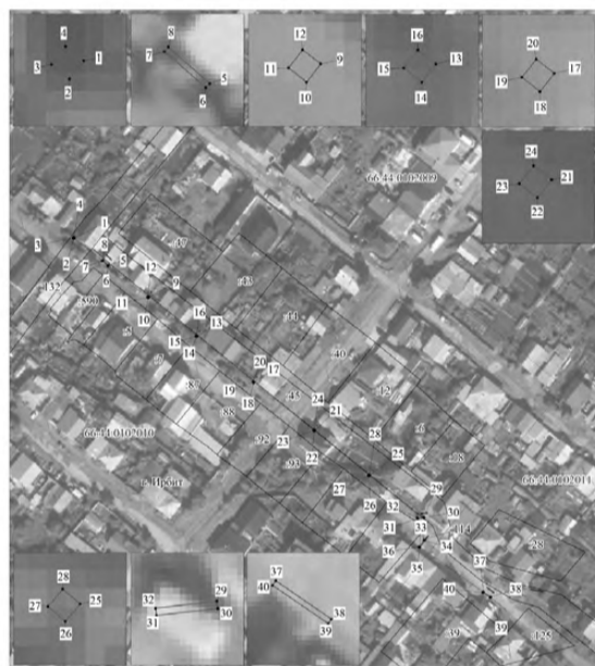
Публичный сервитут ВЛ-6 кВ на деревянных опорах с ж/б приставками от ТП 3104 до ТП 3105 Схема расположения границ публичного сервитута
