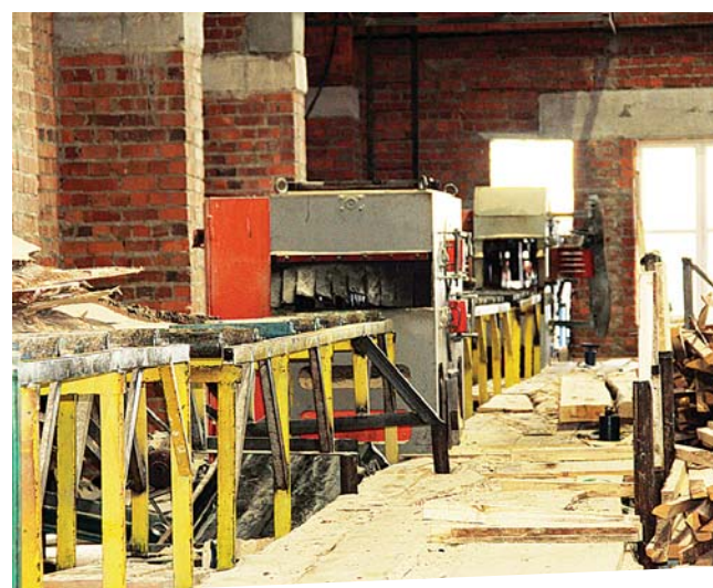
Процесс ленточного распила бревна
