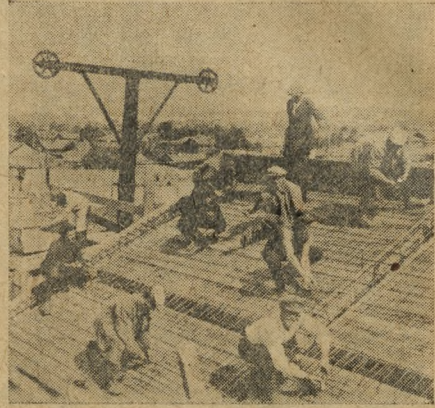
На снимке:—Вяжут переплет для цементирования крыши. Под'емник подает шлак для цементирования.
