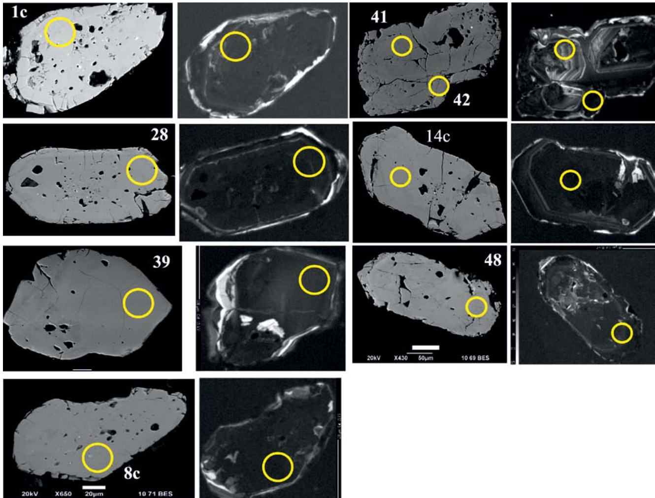
Рис. 1. Оптические (слева) и катодоллюминесцентные (справа) изображения цирконов из гранитов битимского комплекса.
