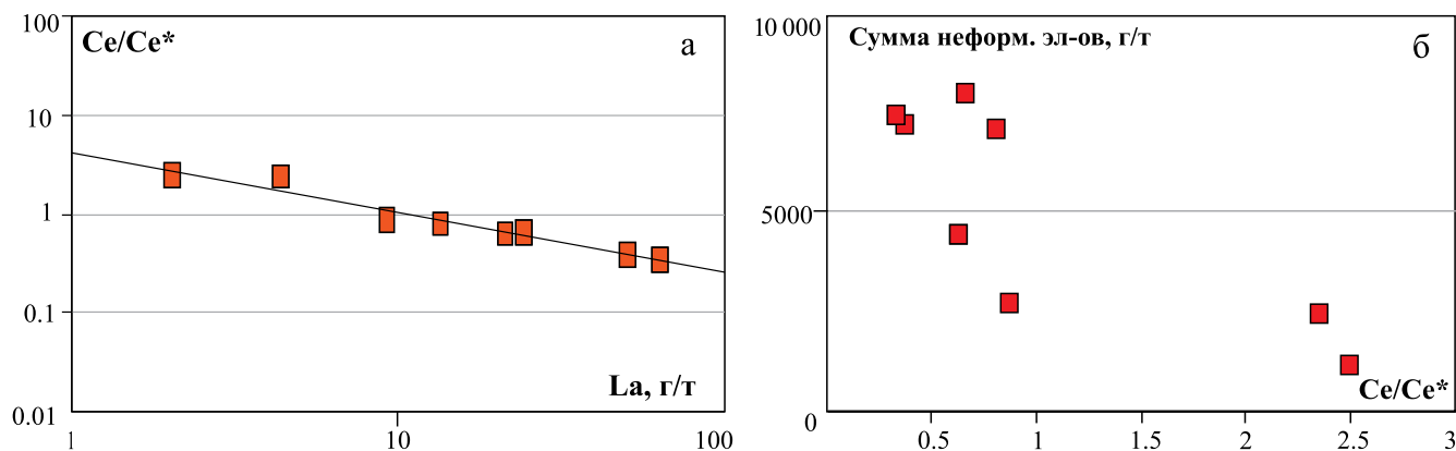
Рис. 4. Диаграмма соотношений La–Ce/Ce* (а), суммы неформальных элементов (включая РЗЭ) и величины аномалии церия (б) для цирконов БГ.
