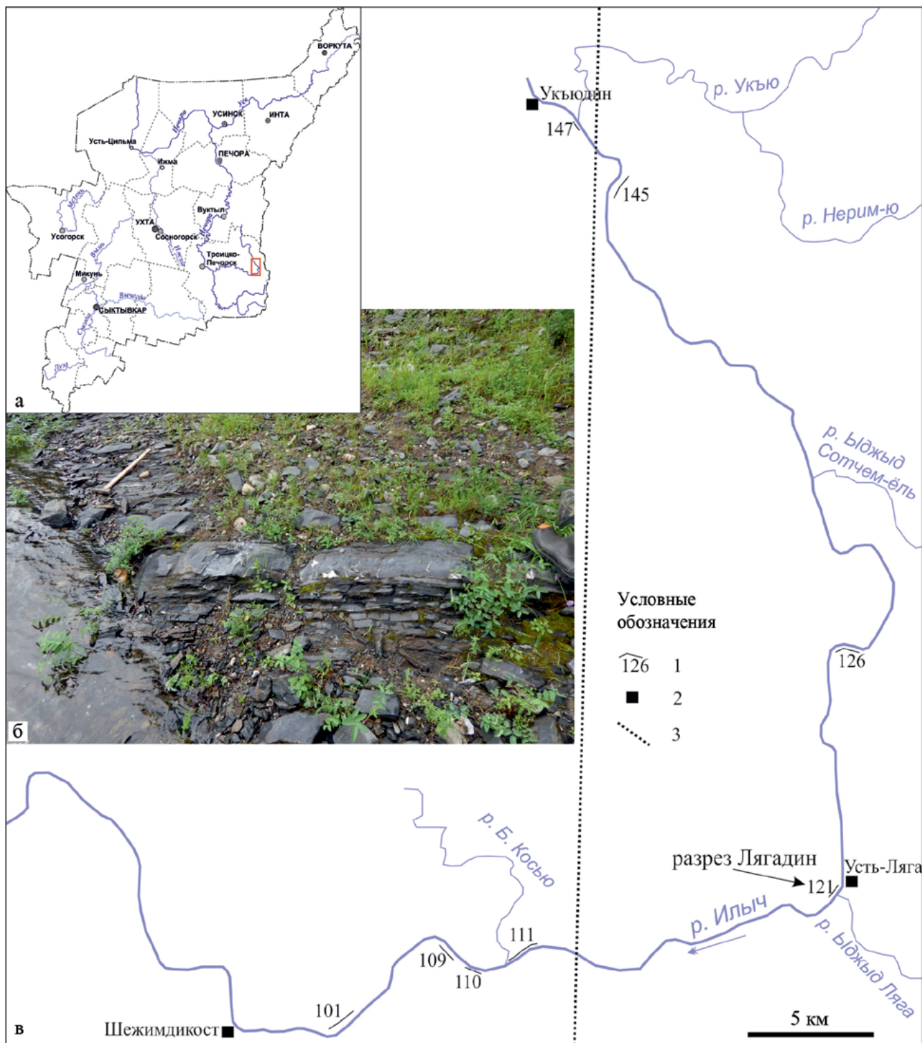
Рис. 1. а. Изученный район на географической карте Республики Коми, РФ. б. Характер выходов нижнелудфордских склоновых отложений в разрезе Лягадин. в. Основные выходы верхнесилурийских разнофациальных отложений на р. Илыч.
