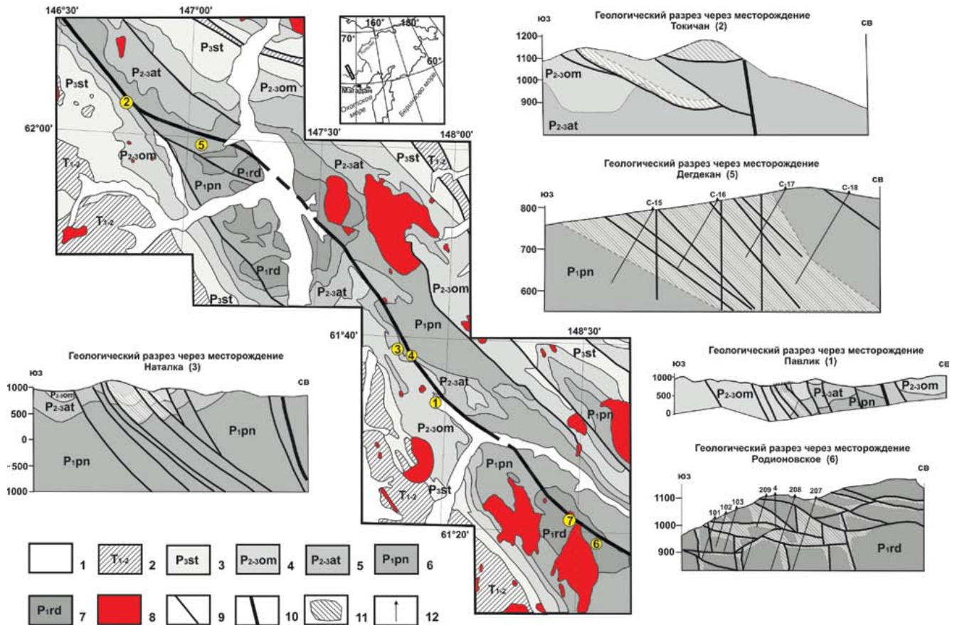
Рис. 1. Схема геологического строения вдоль Тенькинского глубинного разлома (составлена на основе Государственной геологической карты масштаба 1 : 500 000) и разрезы через месторождения золота. На врезке – положение рассматриваемого региона.
