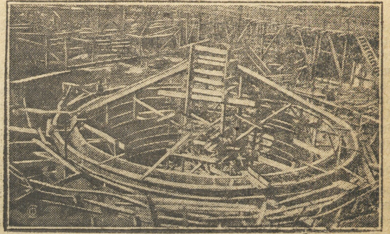
На Краматорском металлургическом заводе (Донбасс) начата стройка новой домны № 4. На снимке: Скиповое кольцо домны № 4.
